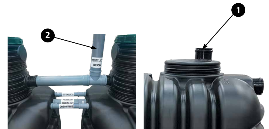
Rysunek 3. Podłączenie rewizji wlotu (1) i wentylacji wysokiej (2)
