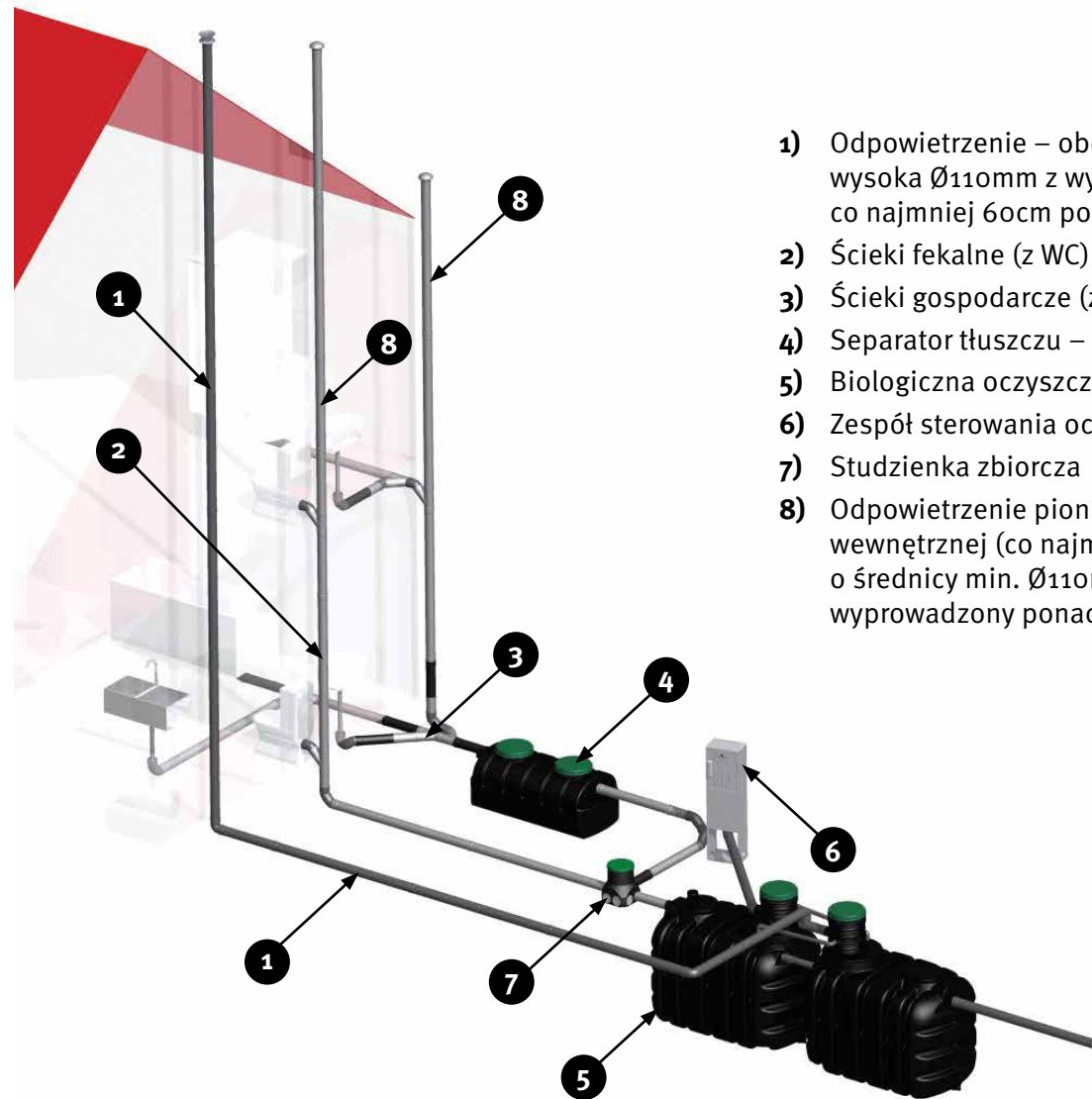
Rysunek 1. Montaż oczyszczalni actibio.
